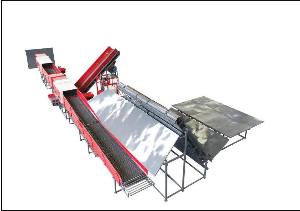
6CZZ-10 型甘蔗除杂设备
